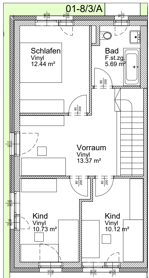
Obergeschoss
