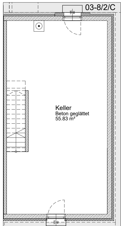
Kellergeschoss
