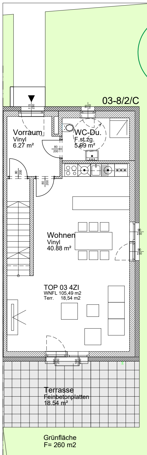
Erdgeschoss
