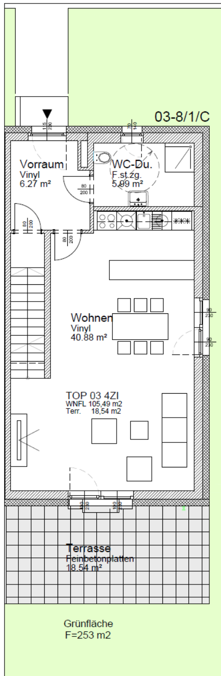
Erdgeschoss
