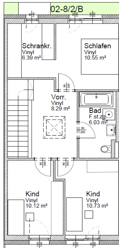
Obergeschoss
