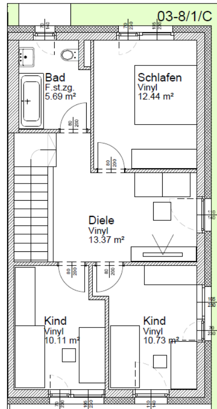
Obergeschoss
