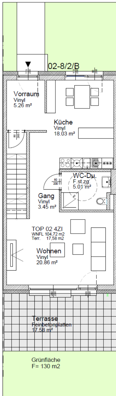
Erdgeschoss
