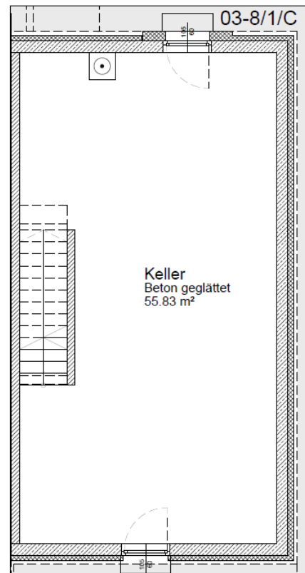
Kellergeschoss
