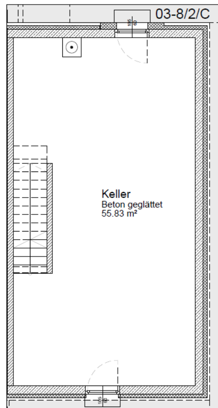
Kellergeschoss
