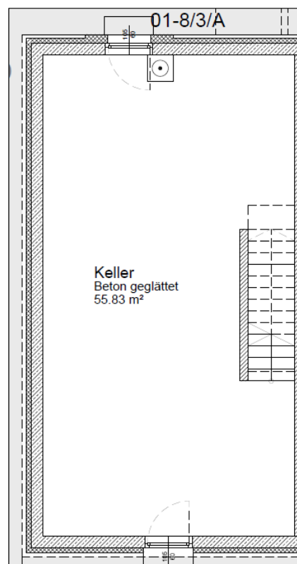
Kellergeschoss
