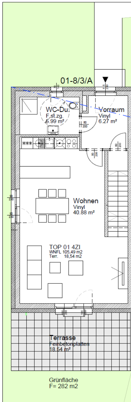
Erdgeschoss
