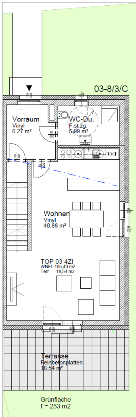
Erdgeschoss
