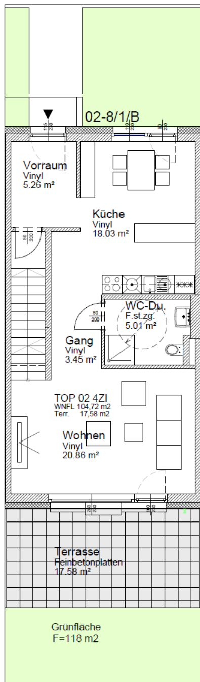
Erdgeschoss
