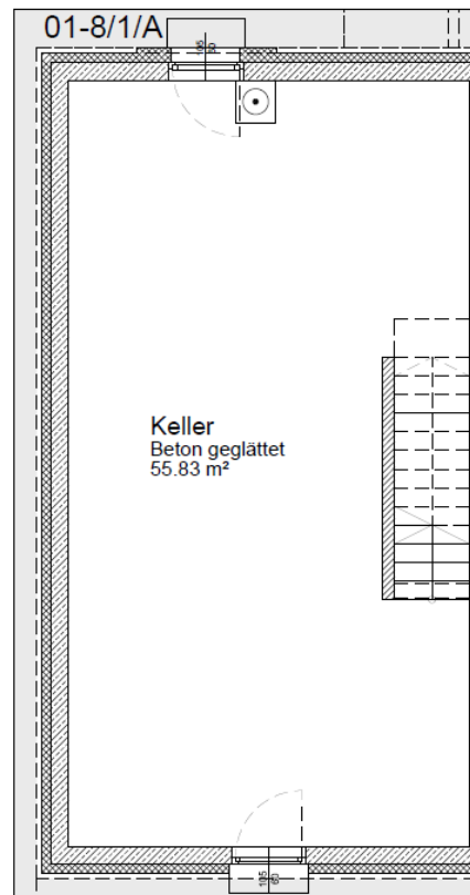
Kellergeschoss
