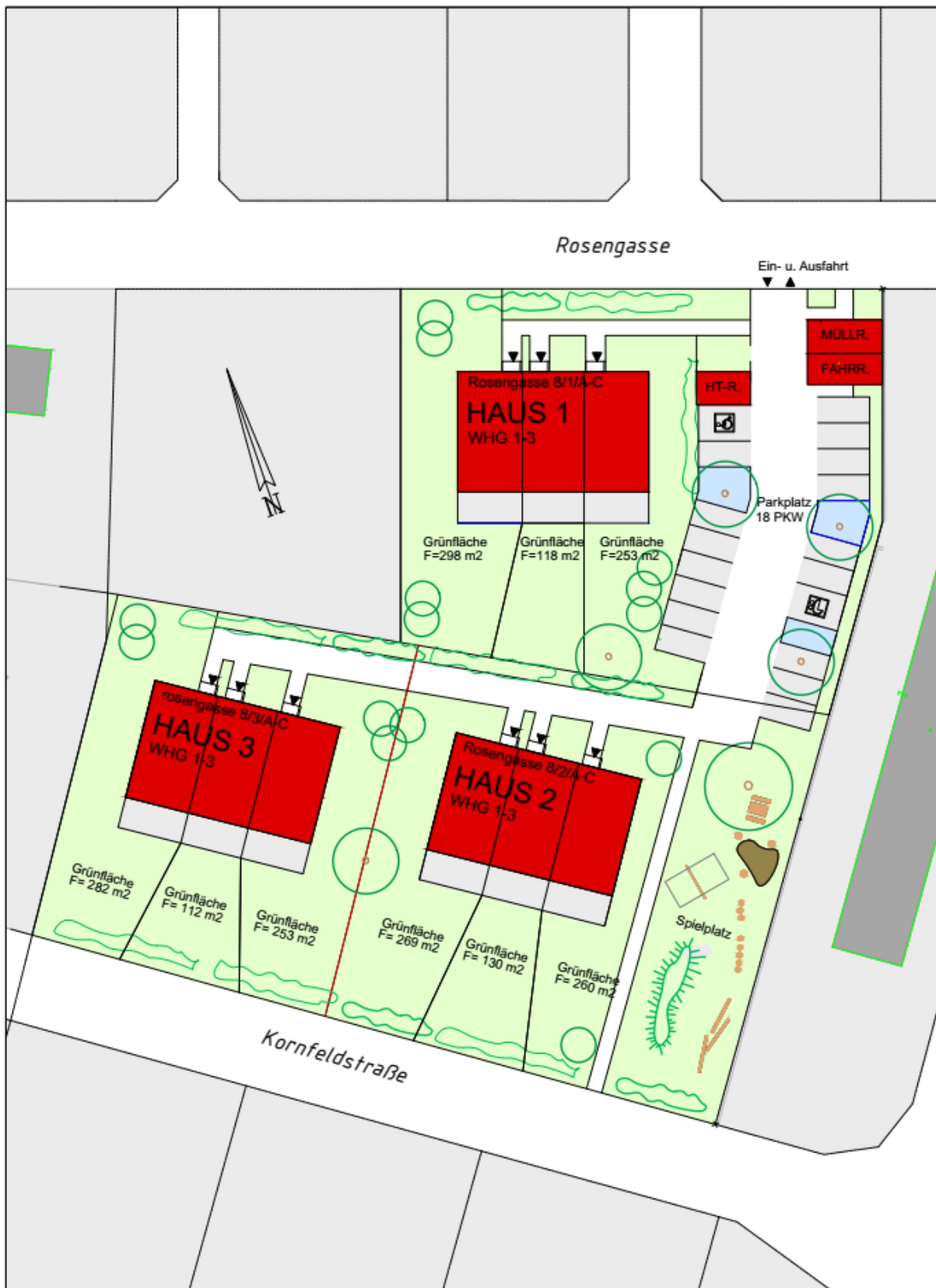
Lageplan M 1 : 500
