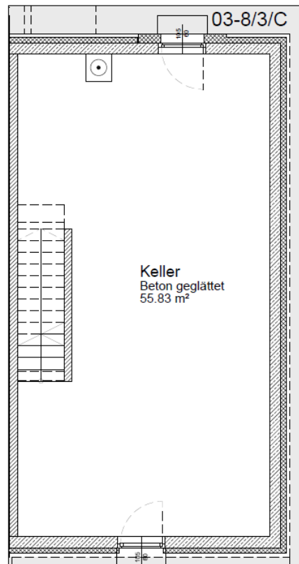
Kellergeschoss
