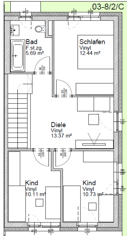
Obergeschoss
