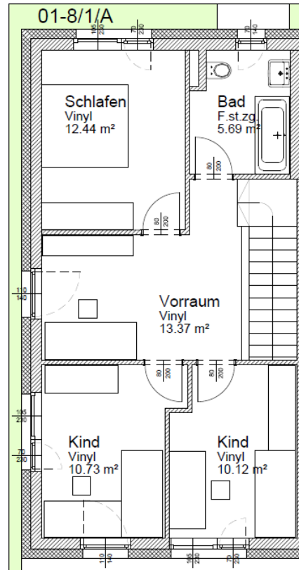
Obergeschoss
