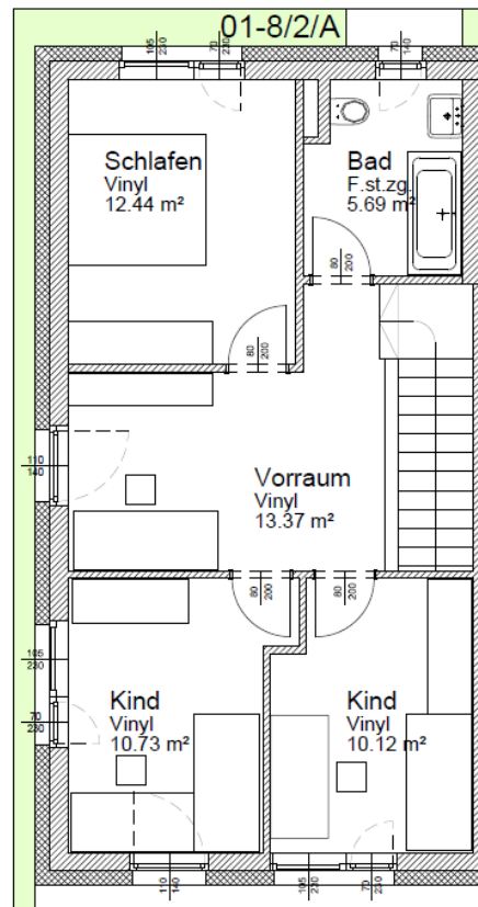
Obergeschoss
