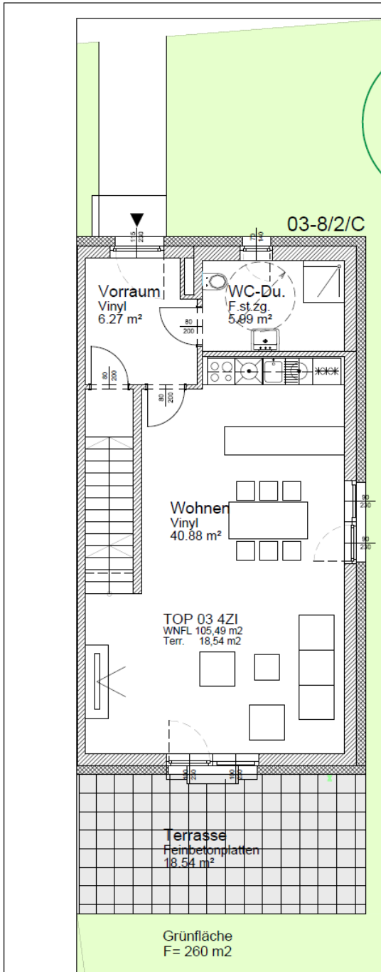
Erdgeschoss
