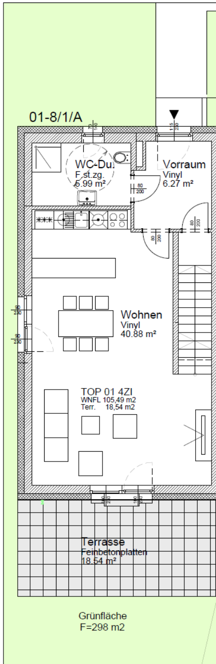
Erdgeschoss
