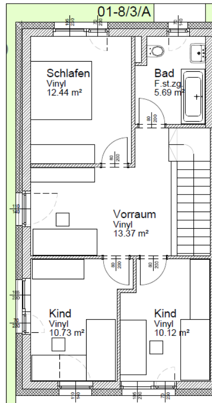
Obergeschoss
