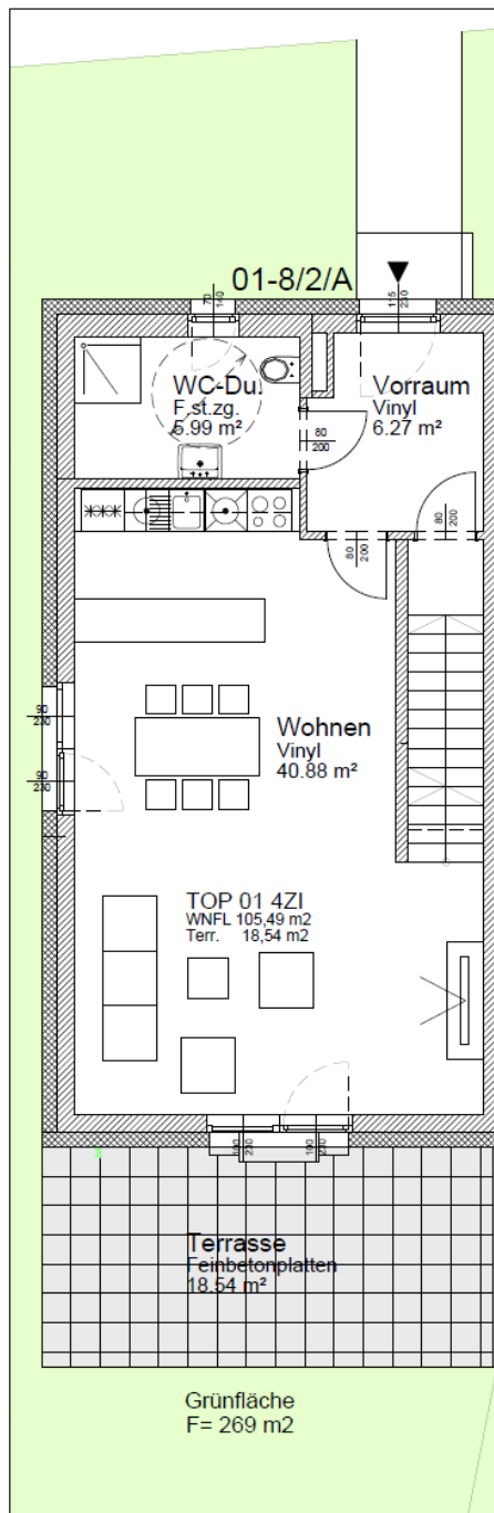
Erdgeschoss
