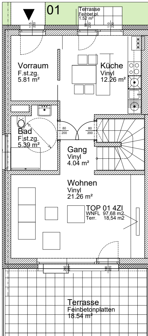
Erdgeschoss
