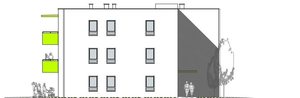
Ansicht Nord-Ost
