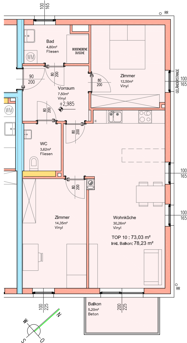
GRUNDRISS 1:100
