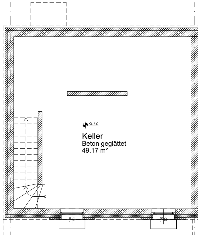
Kellergeschoß
