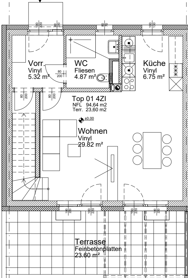
Erdgeschoß
